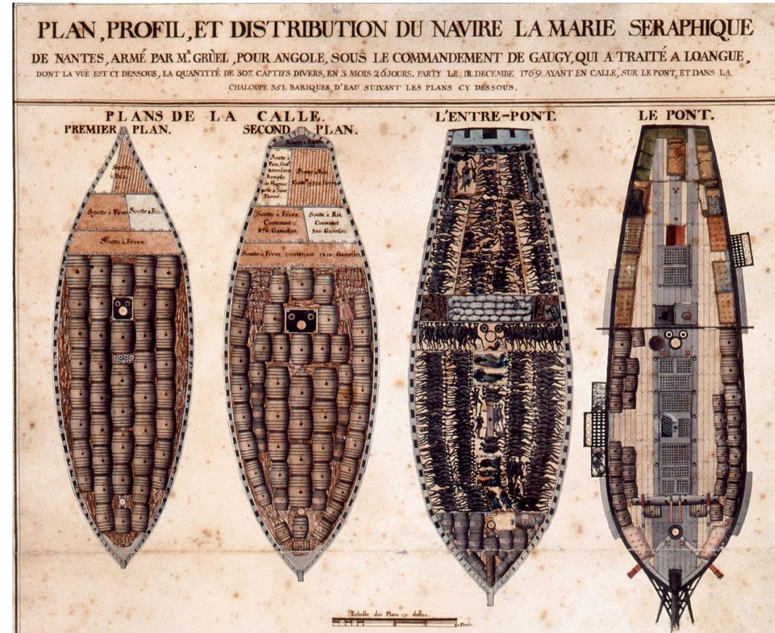
PLAN D'UN NAVIRE NÉGRIER DE NANTES, TRAITE D'AOÛT À DÉCEMBRE 1769. LES ESCLAVES VENANT D'ANGOLA SONT ENTASSÉS SUR L'ENTRE-PONT.
